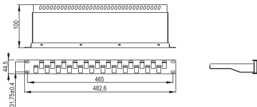
Рисунок / Figure 2 – PP24-1UMU-D
