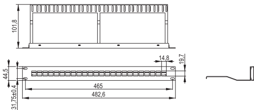
Рисунок / Figure 1 – PP24-1UMU
