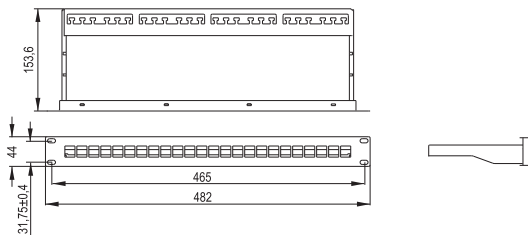
Рисунок / Figure 3 – PP24-1UMF
