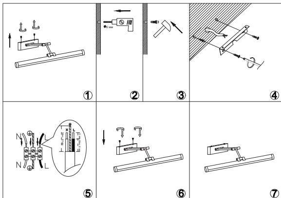
Рисунок 5 — Схема монтажа светильника типа 5115
