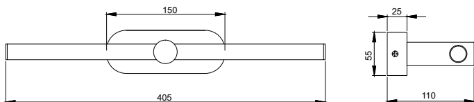
Рисунок 1 — Габаритные размеры светильника типа 5114
