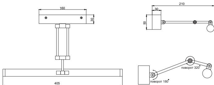
Рисунок 2 — Габаритные размеры светильника типа 5115
