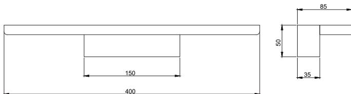
Рисунок 3 — Габаритные размеры светильника типа 5116
