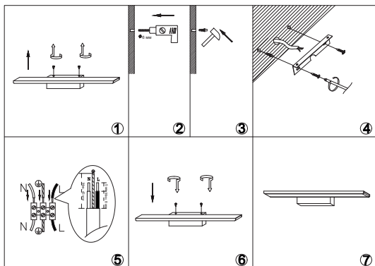
Рисунок 6 — Схема монтажа светильника типа 5116
