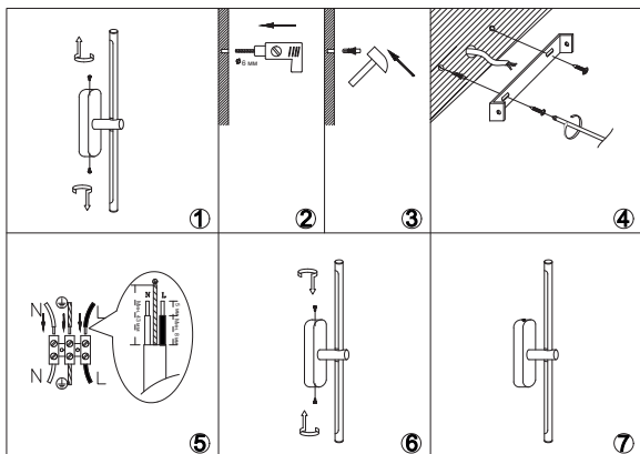
Рисунок 4 — Схема монтажа светильника типа 5114
