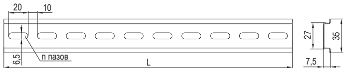
Рисунок 1 — DIN-рейка. Общий вид
