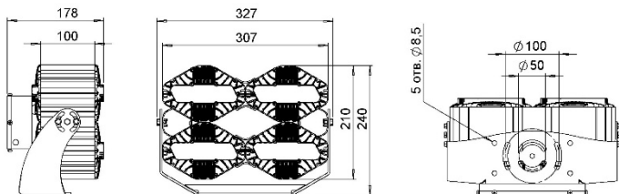
Рисунок 1 Общий вид светильника «L-lego II 220 banner» Поворотное крепление
