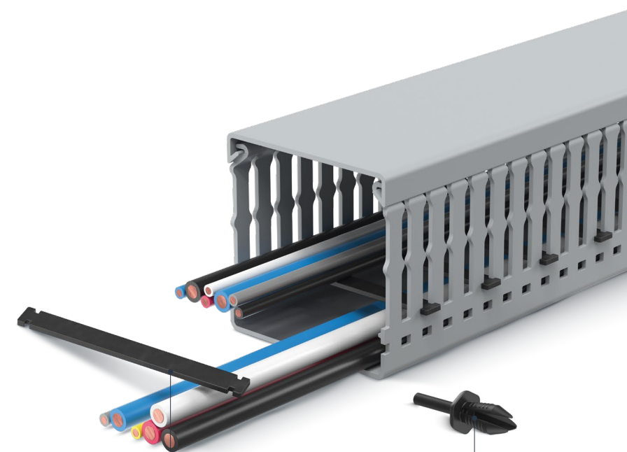
Фиксатор (заклепка)
