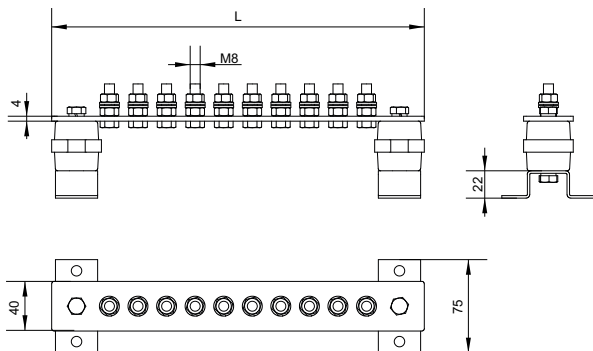
Рисунок / Figure 1 – Габаритные размеры / Overall dimensions
