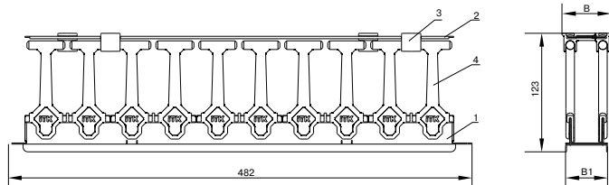
Рисунок 1 – Кабель-органайзер (1 – основание, 2 – крышка, 3 – скрепка, 4 – стойка) / Figure 1. Cable organizer (1 – base, 2 – cover, 3 – clip, 4 – rack)
