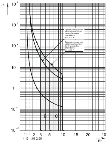
Времятоковые характеристики выключателей / Time-current characteristics of RCBO
