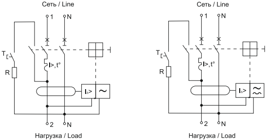
а) АВДТ типа АС / RCBO type AC
