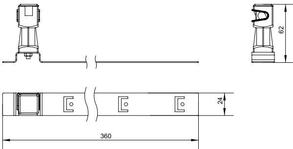
Рисунок / Figure 1 – Габаритные размеры / Overall dimensions
