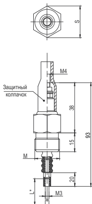
Рисунок 1 – Габаритные и установочные размеры датчика
