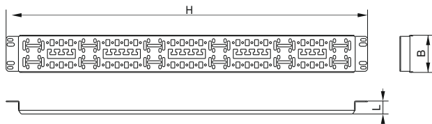
Рисунок 4 – Внешний вид органайзера кабельного горизонтального / Figure 4 – Appearance of the horizontal cable organizer / 4-сурет – Көлбеу кабель органайзерінің сыртқы көрінісі
