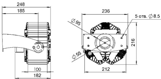
Рисунок 1 Общий вид светильника «L-lego II 165 banner» Поворотное крепление
