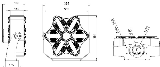
Рисунок 1 Общий вид светильника «L-lego II 330 banner» Поворотное крепление
