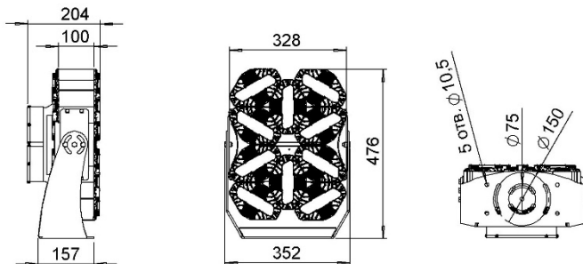
Рисунок 1 Общий вид светильника «L-lego II 500 banner» Поворотное крепление
