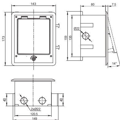
Рисунок / Figure / Сурет 5 – Лючок напольный с ключом на 3 или 6 модулей / Floor box with key, for 3 or 6 modules / 3 немесе 6 модульге арналған кілтті еден люгі (PMLN12-03-K-66-K[XX], PMLN12-06-K-66-K[XX])
