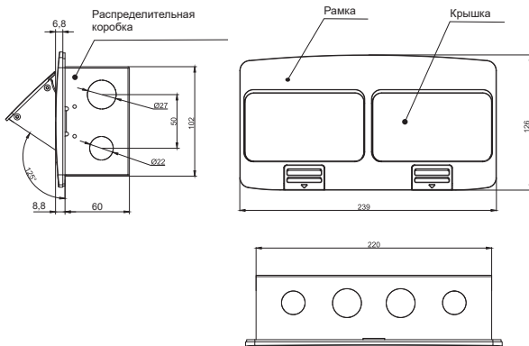
Рисунок / Figure / Сурет 11 – Лючок с откидной крышкой на 6 модулей / Box with flip-up lid, for 6 modules / 6 модулге арналған қайырмалы қақпағы бар люк РМ-LN21-03-О-44-К[XX]
