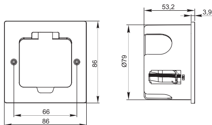
Рисунок / Figure / Сурет 2 – Лючок в фальшпол / Box for raised floor / Фальшеденге арналған люк (PM-LN33-02-O-44-K[XX])
