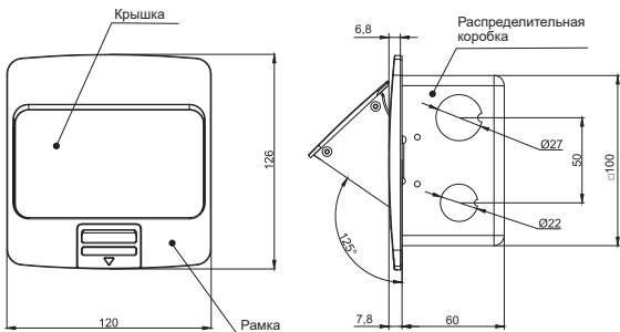
Рисунок / Figure / Сурет 10 – Лючок с откидной крышкой на 3 модуля / Box with flip-up lid, for 3 modules / 3 модульге арналған қайырмалы қақпағы бар люк PM-LN21-03-O-44-K[XX]
