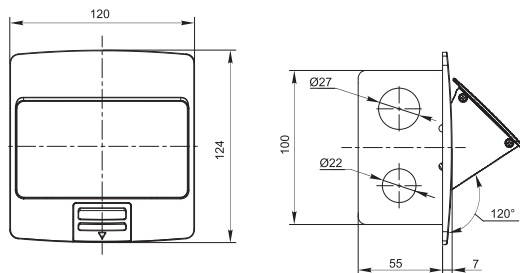
Рисунок / Figure / Сурет 6 – Лючок с откидной крышкой на 3 модуля / Box with flip-up lid, for 3 modules / 3 модульге арналған қайырмалы қақпағы бар люк (PM-LN21-03-O-42-K[XX])
