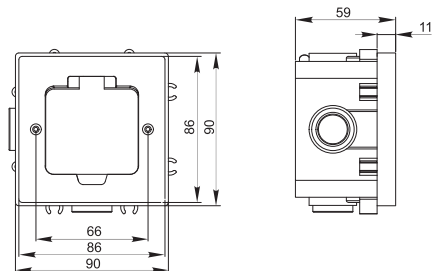
Рисунок / Figure / Сурет 1 – Лючок в бетонный пол / Box for concrete floor / Бетон еденге арналған люк (PM-LN43-02-O-44-K[XX])
