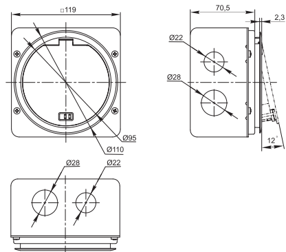
Рисунок / Figure / Сурет 3 – Лючок круглый на 3 модуля / Round box for 3 modules / 3 модульге арналған дөңгелек люк (PM-LN12-03-O-65-K[XX])
