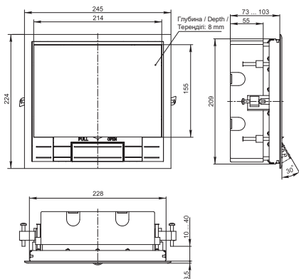
Рисунок / Figure / Сурет 8 – Лючок напольный 12 модулей / Floor box for 12 modules / 12 модульге арналған еден люгі (PM-LN12-12-O-20-K[XX], PMLN1412-O-20-K[XX])
