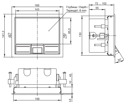
Рисунок / Figure / Сурет 7 – Лючок напольный 8 модулей / Floor box for 8 modules / 8 модульге арналған еден люгі (PM-LN12-08-O-20-K[XX])
