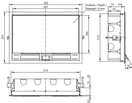
Рисунок / Figure / Сурет 9 – Лючок напольный 16 или 24 модуля / Floor box for 16 or 24 modules / 16 не 24 модульге арналған еден люгі (PM-LN12-16-O-20-K[XX], PM-LN12-24-O-20-K[XX])
