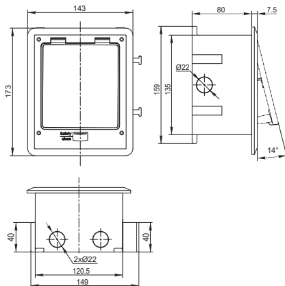
Рисунок / Figure / Сурет 4 – Лючок напольный с кнопкой на 3 или 6 модулей / Floor box with push-button, for 3 or 6 modules / 3 немесе 6 модульге арналған түймешікті еден люгі (PM-LN12-03-B-66-K[XX], PM-LN12-06-B-66-K[XX])
