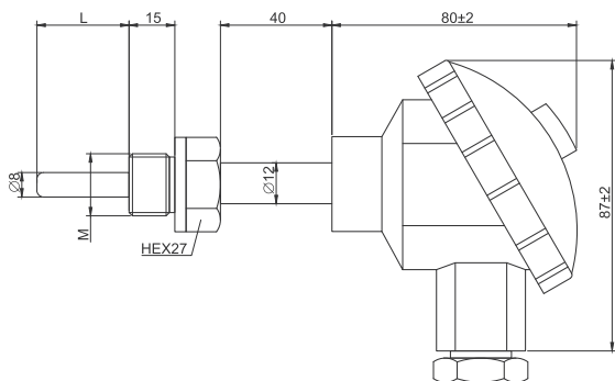
б) преобразователь погружной с монтажной головкой (PTS-X-X-X-4-X-X)
