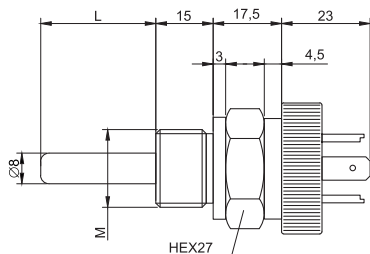
а) преобразователь погружной с присоединением DIN43650 (PTS-X-X-X-2-X-X)
