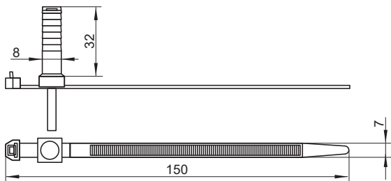
Рисунок 1 – Габаритные размеры хомута / Figure 1 – Clip overall dimensions
