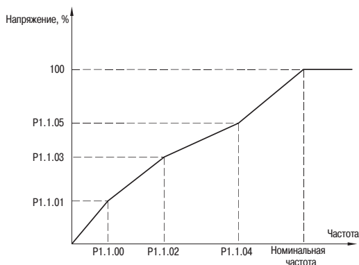
Рисунки 31 – Произвольная кривая V/F
