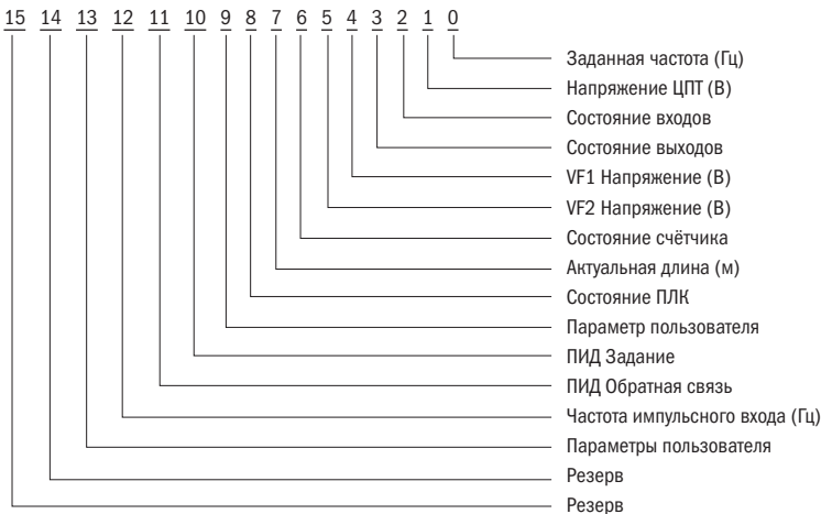
Рисунок 43 – Отображение LED при остановке
