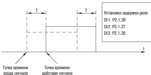
Рисунок 77 – Задержка срабатывания времени T
