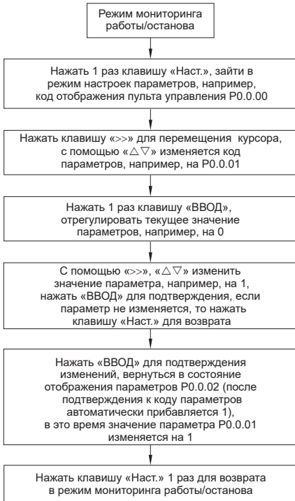
Рисунок 22 – Настройка параметров с помощью пульта управления
