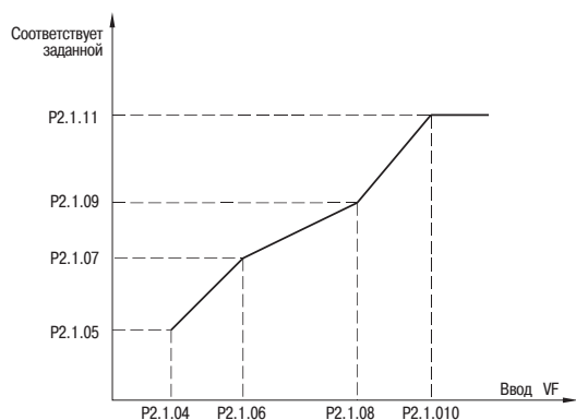
Рисунок 32 – Произвольная кривая 3 аналогового входа
