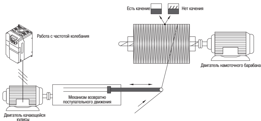
Рисунок 73 – Пример оборудования для использования частоты колебания
