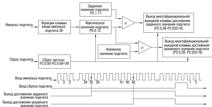
Рисунок 61 – Работа функции подсчёта
