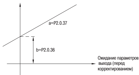
Рисунок 76 – Настройка аналогового выхода
