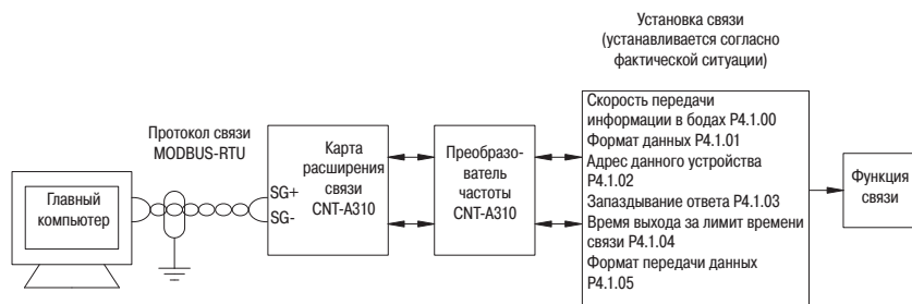
Рисунок 79 – Соединение по интерфейсу с внешним PLC
