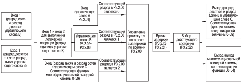
Рисунок 63 – Программирование промежуточного реле
