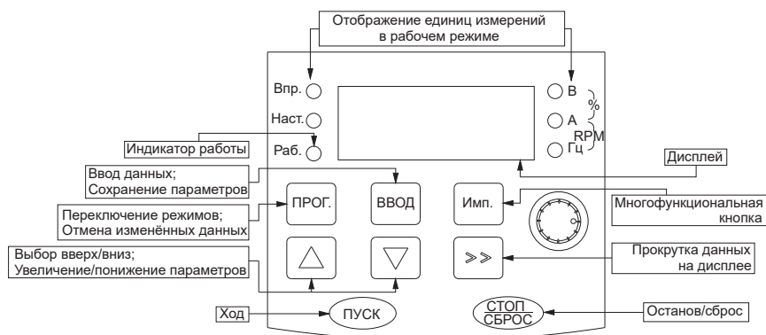
Рисунок 18 – Пульт управления преобразователем частоты
