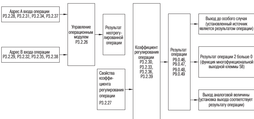
Рисунок 71 – Работа операционного модуля
