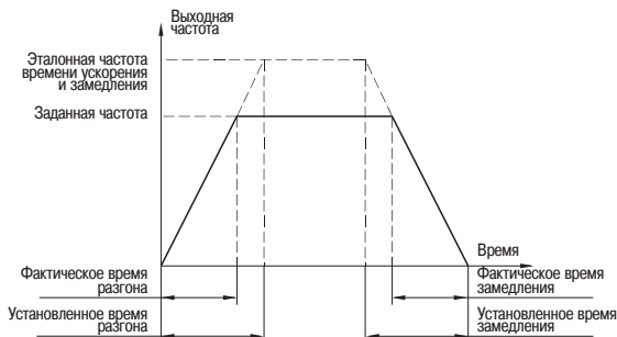
Рисунок 24 – Время ускорения и замедления
