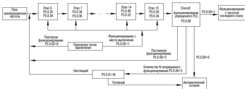
Рисунок 58 – Работа с упрощённым PLC
