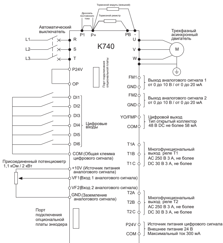
Рисунок 12 – Схема силовой цепи и контура управления преобразователя частоты K740
