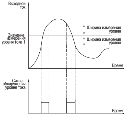
Рисунок 38 – Измерение уровня тока
