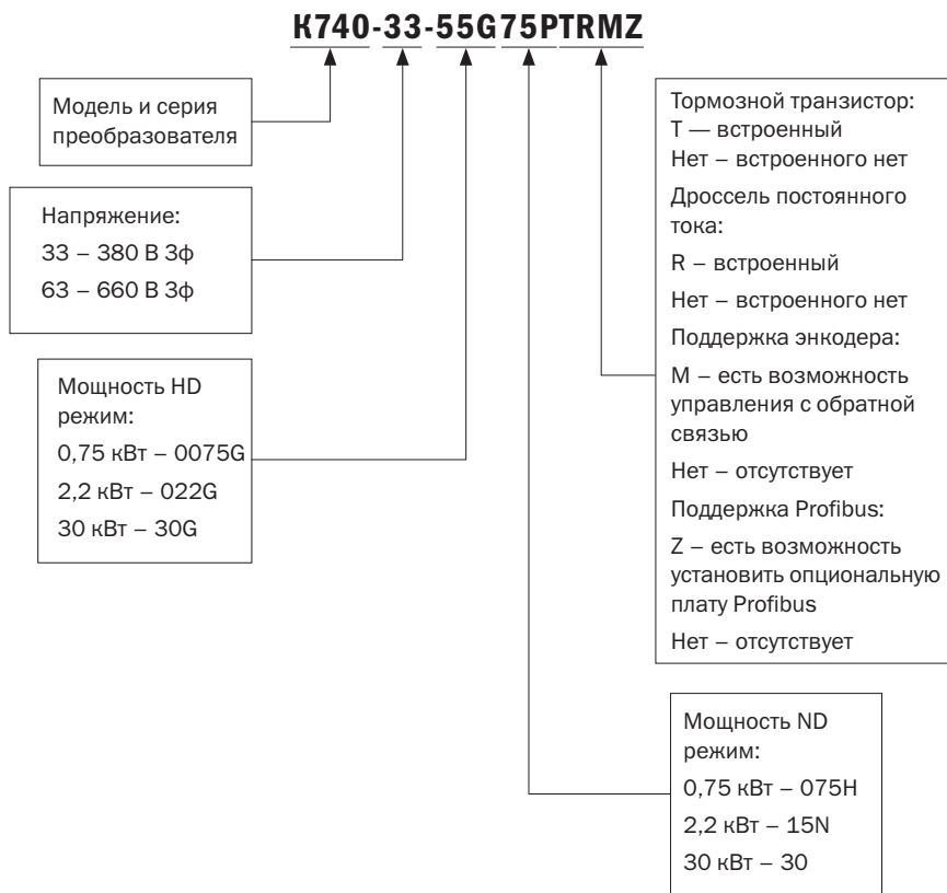
Рисунок 1 – Пример расшифровки артикула преобразователя частоты
