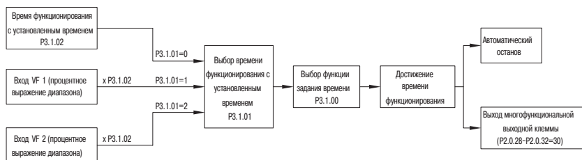
Рисунок 59 – Работа функции контроля времени
