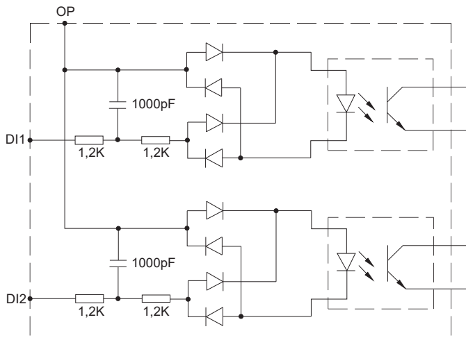
Рисунок 13 – Схема цифровых входов
