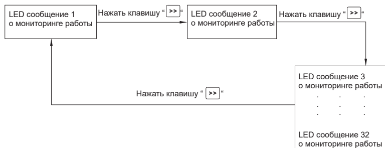
Рисунок 21 – Просмотр состояния преобразователя в остановленном состоянии
