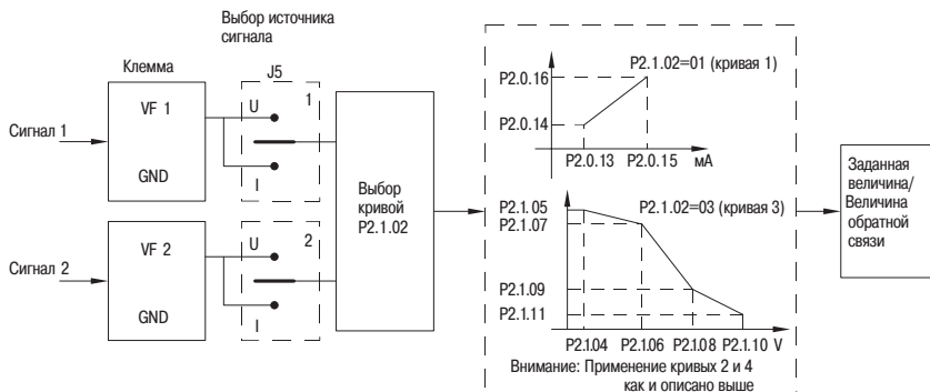
Рисунок 75 – Настройка аналоговых входов
