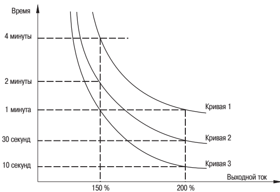
Рисунок 30 – Кривые защиты от перегрузки
