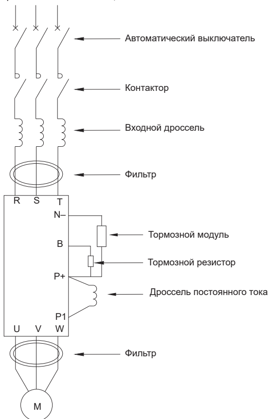
Рисунок 8 – Подключение периферийных устройств
