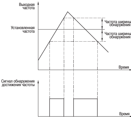
Рисунок 33 - Ширина обнаружения заданной частоты
