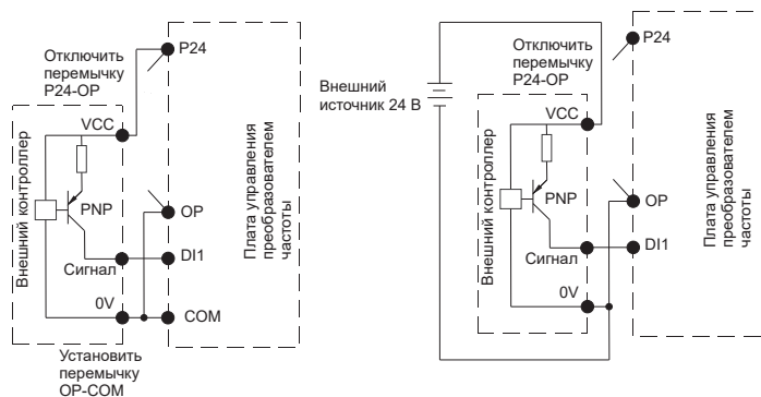
г) цифровые выходы ПЛК PNP (источник)
