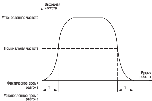
Рисунок 25 – S кривая ускорения и замедления
