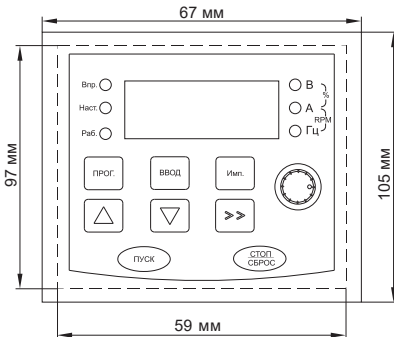
Рисунок 19 – Габаритные размеры пульта управления
