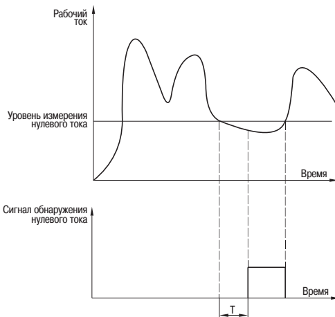
Рисунок 36 – Измерение нулевого тока
