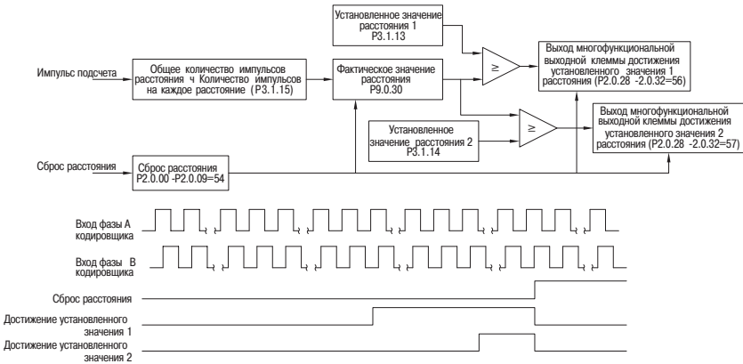
Рисунок 62 – Работа функции контроля расстояния
