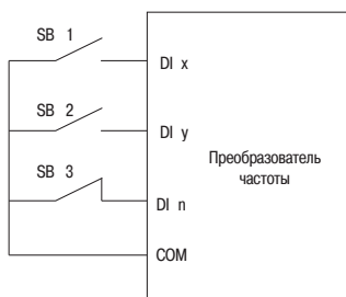
Рисунок 49 – Трёхпроводной способ управления 1
