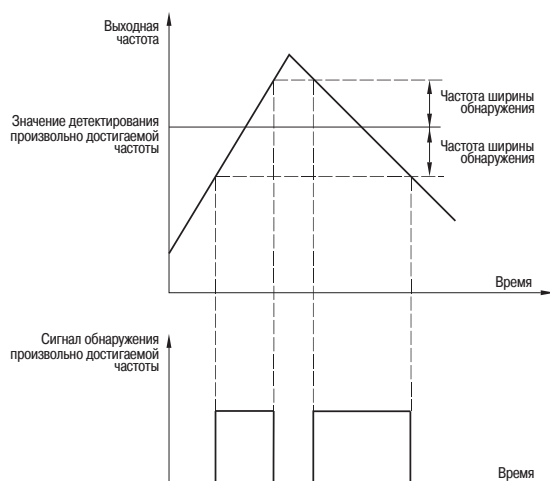
Рисунок 35 - Произвольно достигаемая частота
