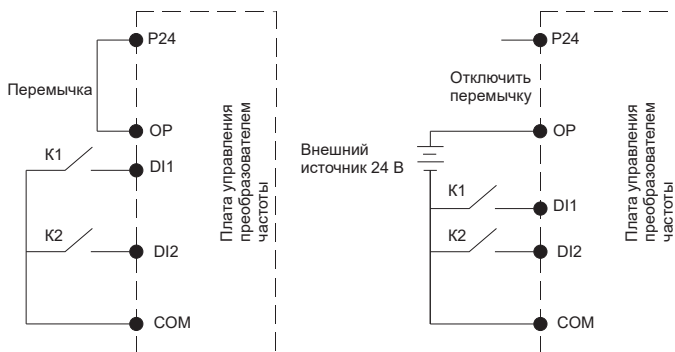
Рисунок 14 – Схемы подключения цифровых входов (лист 1 из 2)
