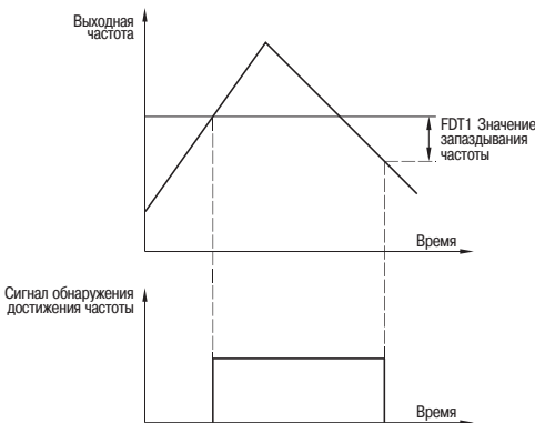
Рисунок 34 - Измерение частоты FDT1
