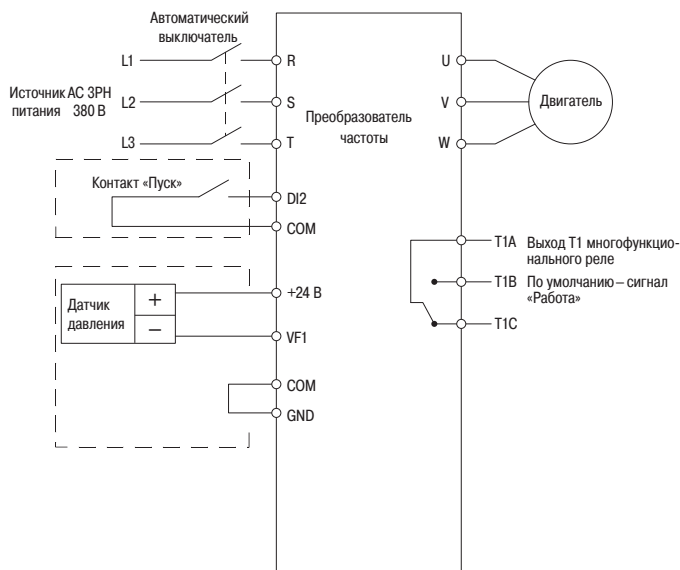
Рисунок 80 – Схема подключения преобразователя частоты для поддержания давления с датчиком с сигналом 4-20 мА
