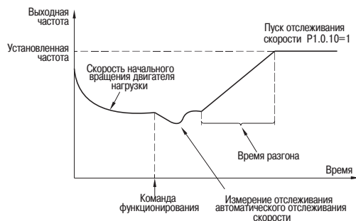
Рисунок 52 – Пуск с поиском скорости
