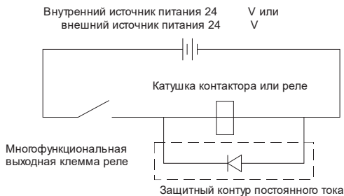
Рисунок 16 – Схема подключения выходного реле на постоянный ток
