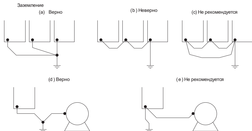
Рисунок 17 – Подключение контура заземления
