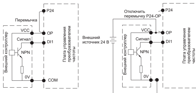
в) цифровые выходы ПЛК NPN (приёмник)
