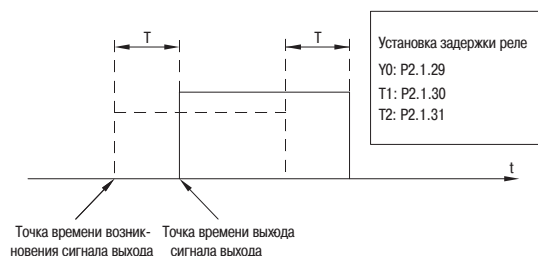
Рисунок 78 – Задержка срабатывания выходного реле
