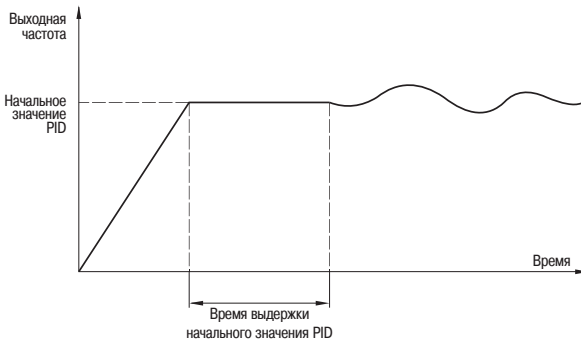
Рисунок 40 – Начальное значение ПИД
