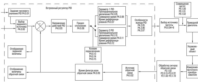
Рисунок 72 – Структура ПИД регулятора
