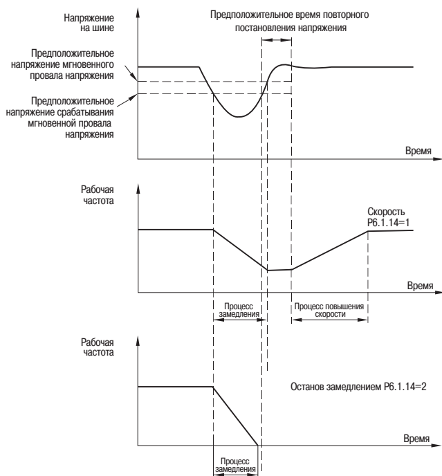
Рисунок 44 – Мгновенное прерывание напряжени
