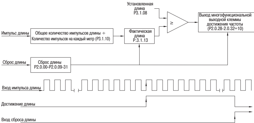
Рисунок 60 – Работа функции контроля длины
