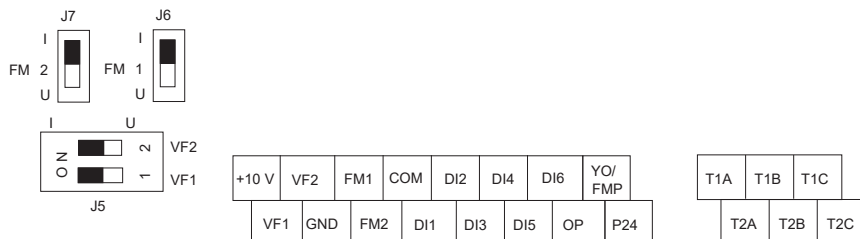
Рисунок 11 – Клеммная колодка преобразователя частоты
