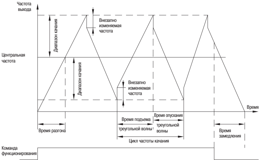
Рисунок 74 – Графики частоты колебания
