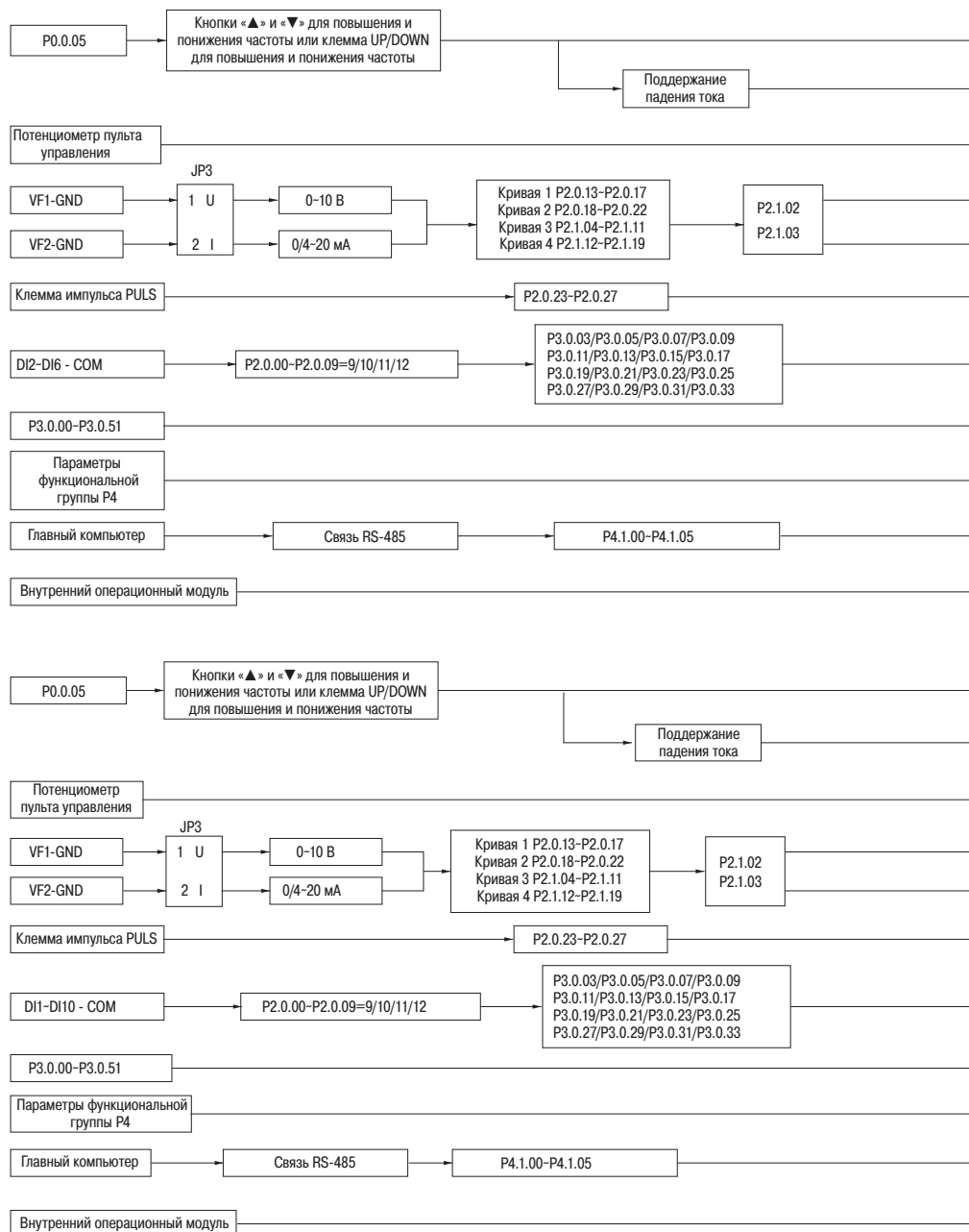
Рисунок 56 - Регулирование частоты вращения
