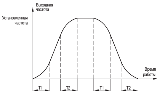
Рисунок 26 – Соотношения S кривых
