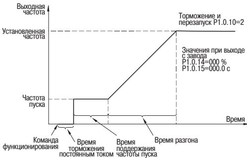
Рисунок 53 – Пуск с торможением постоянным током
