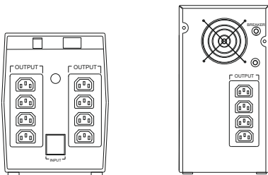
Рисунок 5 – Задняя панель ИБП без коммуникационного порта или с портом USB (опционально) и разъемами С13
