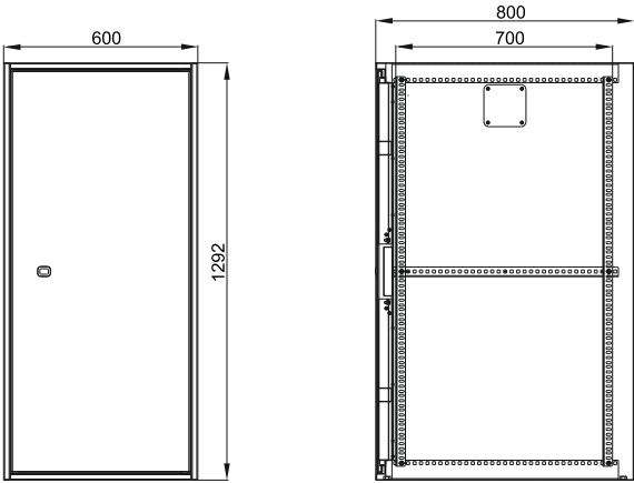
Рисунок 1 – Внешний вид, габаритные и установочные размеры шкафа
