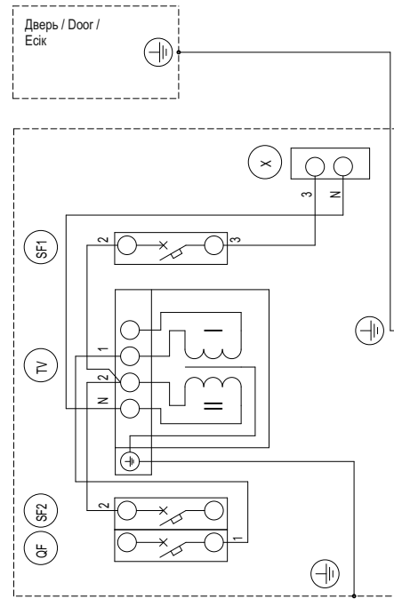
ЯТП-0,25 230/24-3 УХЛ2 IP54
