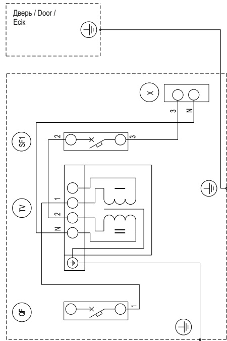
ЯТП-0,25 230/24-2 УХЛ2 IP54
