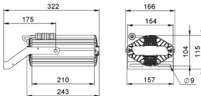
Рисунок 1 Общий вид светильника «L-lego II 30 banner» Поворотное крепление
