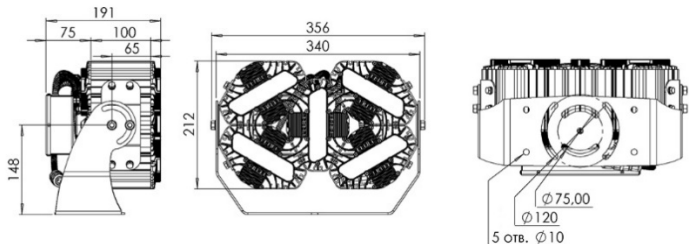
Рисунок 1 Общий вид светильника «L-lego II 250 banner» Поворотное крепление
