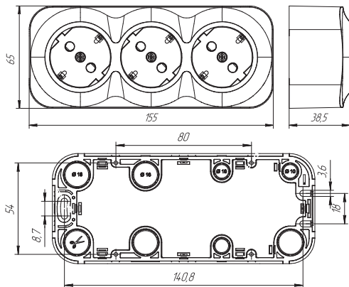
b) Розетка трехместная / Three-gang socket-outlet / Үш орындық розетка / Priză triplă / Uch o'rinli rozetka
