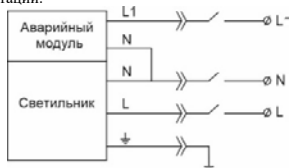
Рисунок 2 Схема подключения светильника
