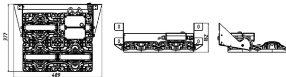
Рисунок 1 Общий вид светильника «L-pixel 4 Em banner» Поворотное крепление
