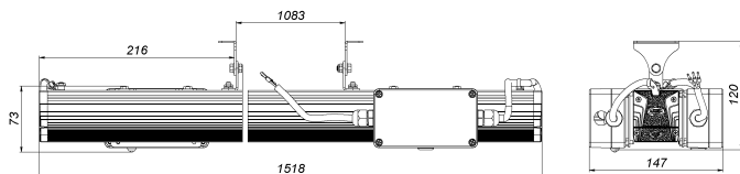
Рисунок 2 Светильник «L-fusion Office/Em» 1,5 м
