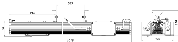
Рисунок 1 Светильник «L-fusion Office/Em» 1,0 м
