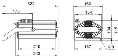
Рисунок 1 Общий вид светильника «L-lego II 55 banner» Поворотное крепление
