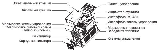
Рисунок 2.1 – Внешний вид и элементы преобразователя
