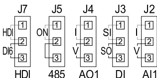
Рисунок 3.11 – Схема перемычек
