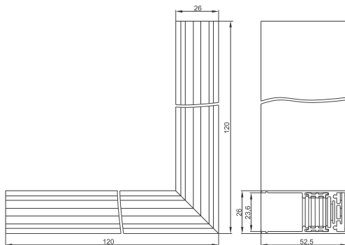
Рисунок 15 – Соединитель L-образный LSB0D-SLNMU-026-K02
