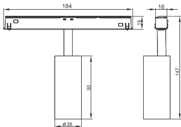
Рисунок 3 – Светильник LT-DSB0-5133-010-26-K02
