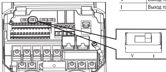
Рисунок 4.4.3. Переключатель AM
