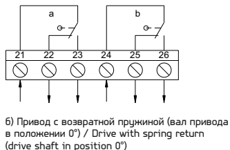
Рисунок 4 – Схемы подключения вспомогательных цепей / Figure 4 – Connection diagrams of auxiliary circuits
