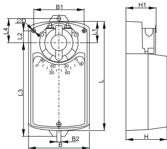
а) Приводы без возвратной пружины / Drive without spring return
