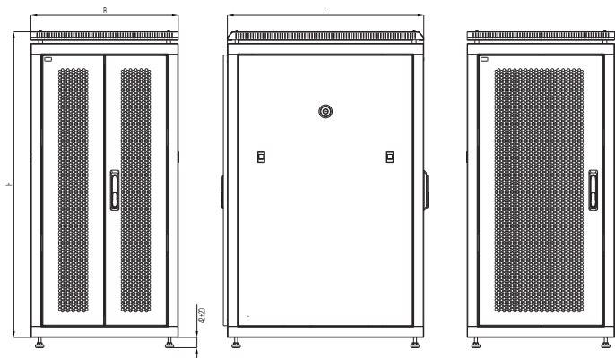
Рисунок 1 – Внешний вид шкафа и габаритные размеры
