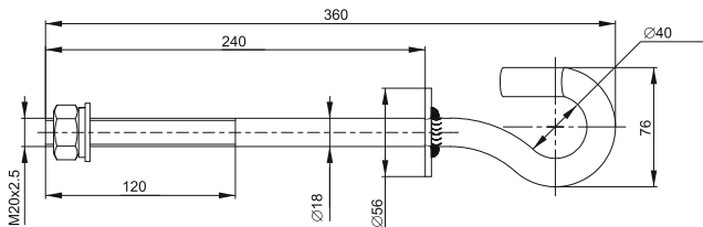
Рисунок 2 – Внешний вид и габаритные размеры крюка монтажного В 20/240 / Figure 2 – Appearance and overall dimensions of mounting hook В 20/240 / 2 сурет – 20/240 В монтаждай ілмегінің сыртқы көрінісі және габариттік өлшемдері
