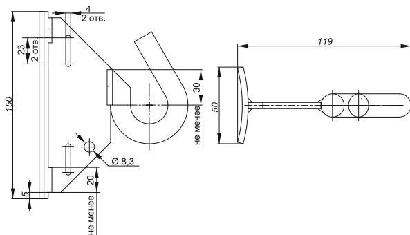
Рисунок 4 – Внешний вид и габаритные размеры крюка монтажного CF 16 / Figure 4 – Appearance and overall dimensions of mounting hook CF 16 / 4 сурет – CF 16 монтаждау ілмегінің сыртқы көрінісі және габариттік өлшемдері
