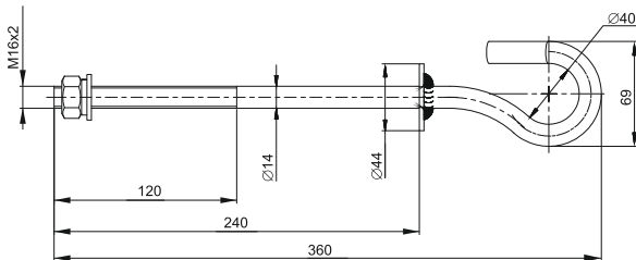
Рисунок 1 – Внешний вид и габаритный размеры крюка монтажного В 16/240 / Figure 1 – Appearance and overall dimensions of mounting hook В 16/240 / 1 сурет – 16/240 В монтаждай ілмегінің сыртқы көрінісі және габариттік өлшемдері
