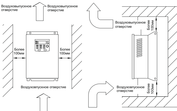
Рисунок 1 – Способ установки преобразователя частоты
