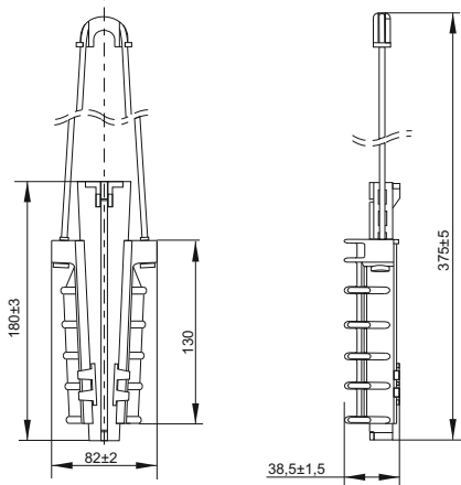
Рисунок 1 – Габаритные и установочные размеры зажима / Figure 1 – Overall and mounting dimensions of the clamp / 1 сурет – Қысқыштың габариттік және орнату өлшемдері
