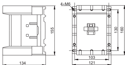
Рисунок 1 – Габаритные и установочные размеры КТИе-5115, КТИе-5150, КТИе-5170 / Figure 1 – Overall and mounting dimensions КТИе-5115, КТИе-5150, КТИе-5170 / 1 сурет – КТИе-5115, КТИе-5150, КТИе-5170 габариттік және орнату өлшемдері
