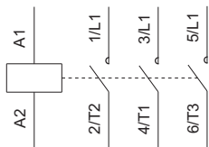
Рисунок 3 – Схема электрическая КТИе-5115, КТИе-5150, КТИе-5170 / Figure 3 – Electric diagram КТИе-5115, КТИе-5150, КТИе-5170 / 3 сурет – КТИе-5115, КТИе-5150, КТИе-5170 электрлі схемасы
