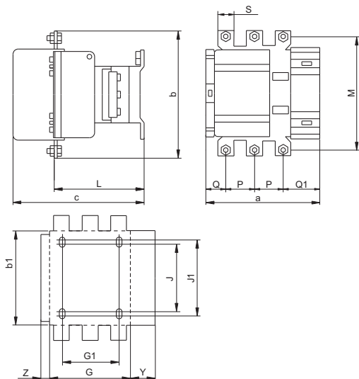
Рисунок 2 – Габаритные и установочные размеры КТІе-5200, КТІе-5250 / Figure 2 – Overall and mounting dimensions КТІе-5200, КТІе-5250 / 2 сурет – КТІе-5200, КТІе-5250 габариттік және орнату өлшемдері
