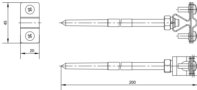
Рисунок / Figure 1 – Габаритные размеры / Overall dimensions
