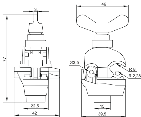
Рисунок 1 – Габаритные размеры ЗОИ / Figure 1 – Overall dimensions of ZOI / 1 сурет – ЗОИ-ның габариттік өлшемдері
