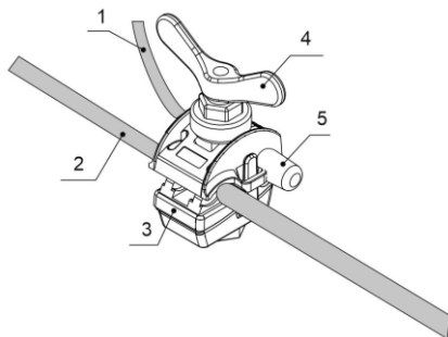
Рисунок 2 – Монтаж ЗОИ / Figure 2 – Installation of the ZOI / 2 сурет – ЗОИ-ны монтаждау
