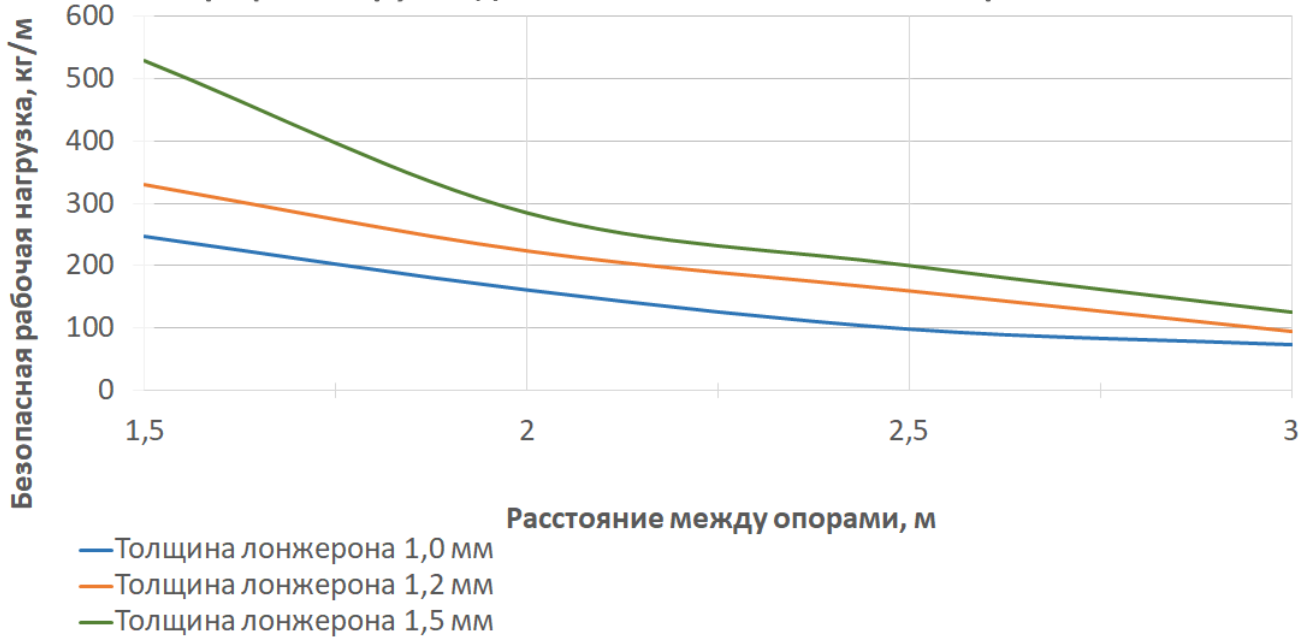
График нагрузок для лотков LESTA с высотой борта 55 мм
