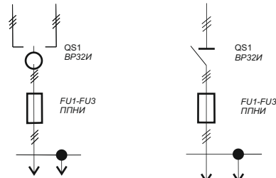
ЯРП на два направления / Power box in two directions / ЯРП екі бағытта
