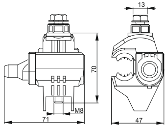
Рисунок 4 – 30И 35-150/6-35
