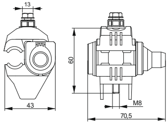
Рисунок 2 – 30И 16-95/2,5-35
