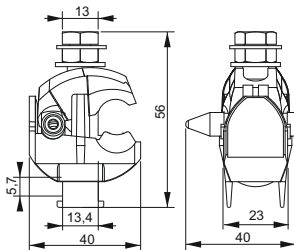
Рисунок 6 – ЗОИ 10-95/1,5-10М
