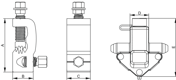
а) ЗОРЗБ-1
