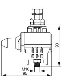
Рисунок 5 – ЗОИ 35-150/35-150
