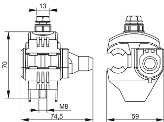
Рисунок 3 – 30И 25-95/25-95
