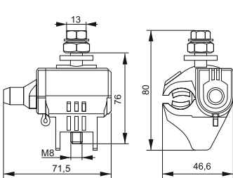
Рисунок 8 – ЗСГП110-95/6-35
