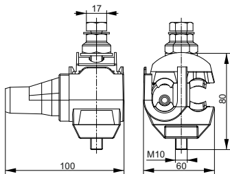
Рисунок 9 – ЗСГП35-120/25-95
