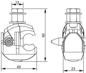
Рисунок 1 – 30И 16-70/1,5-10
