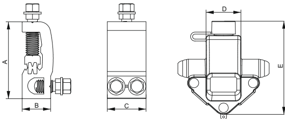
б) ЗОРЗБ-2
