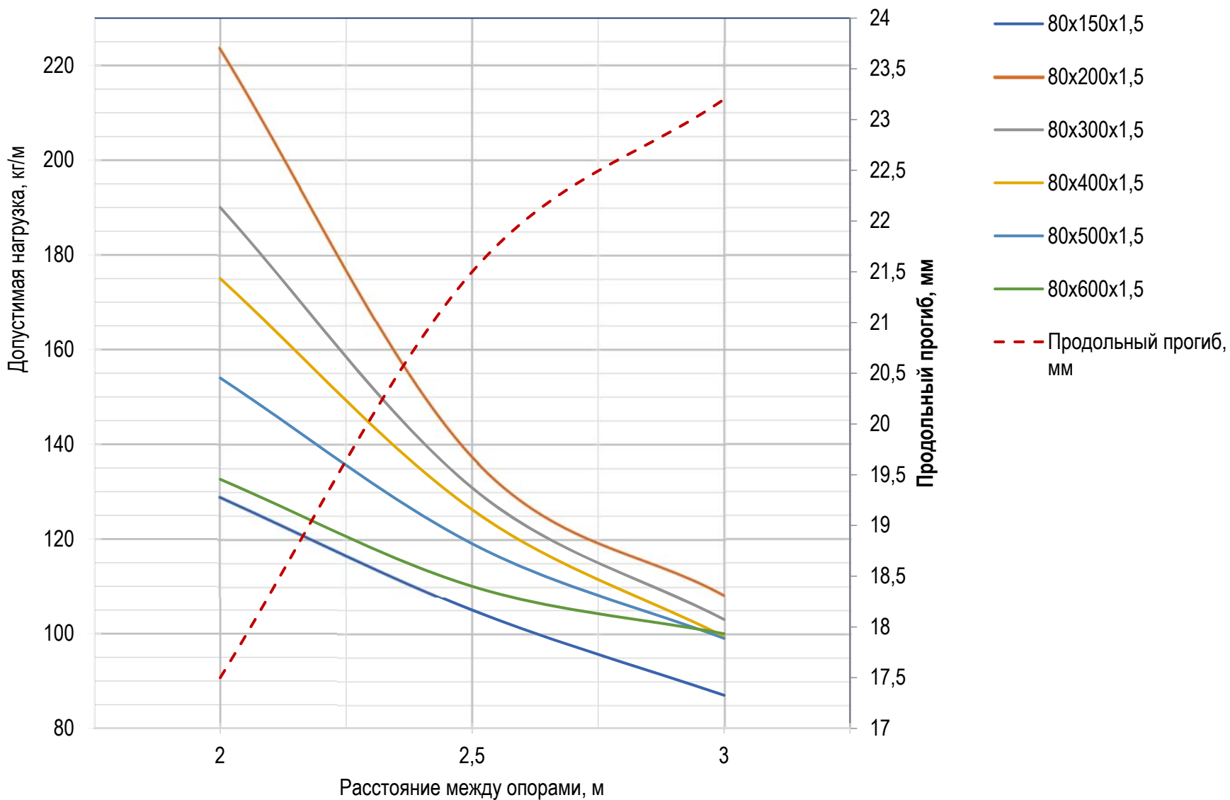
График нагрузок для лотков высотой 80 мм с толщиной стали 1,5 мм
