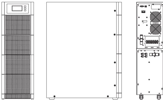
Внешний вид ИБП типа / Appearance of UPS of types / Типті ҮҚК сыртқы көрінісі EOT-0010KVA-1-L, EOT-0010KVA-1-020
