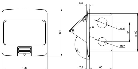
Рисунок / Figure / Сурет 10 — Лючок с откидной крышкой на 3 модуля / Box with flip-up lid, for 3 modules / 3 модульге арналған қайырмалы қақпағы бар люк PM-LN21-03-O-44-K[XX]
