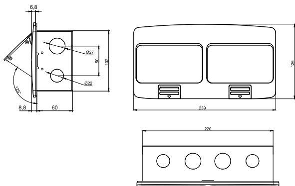
Рисунок / Figure / Сурет 10 — Лючок с откидной крышкой на 3 модуля / Box with flip-up lid, for 3 modules / 3 модульге арналған қайырмалы қақпағы бар люк PM-LN21-03-O-44-K[XX]
