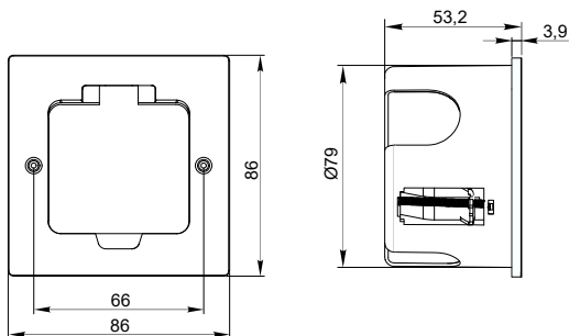
Рисунок / Figure / Сурет 2 — Лючок в фальшпол / Box for raised floor / Фальшденге арналған люк (PM-LN33-02-O-44-K[XX])
