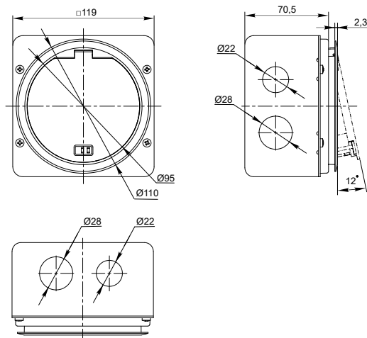
Рисунок / Figure / Сурет 3 — Лючок круглый на 3 модуля / Round box for 3 modules / 3 модульге арналған дөңгелек люк (PM-LN12-03-O-65-K[XX])
