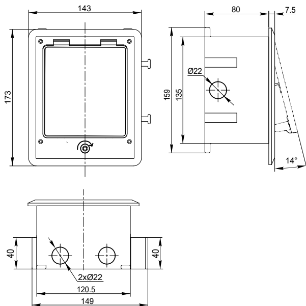
Рисунок / Figure / Сурет 5 — Лючок напольный с ключом на 3 или 6 модулей / Floor box with key, for 3 or 6 modules / 3 немесе 6 модульге арналған кілтті еден люгі (PM-LN12-03-K-66-K[XX], PM-LN12-06-K-66-K[XX])
