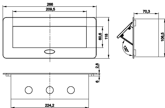
Рисунок 2 — Блок розеточный с выдвижной крышкой 6 модулей (PM-BR51-06-O-KXX)
