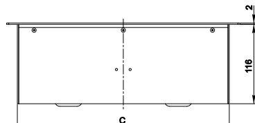
Рисунок 4 — Блок розеточный с двусторонней крышкой
