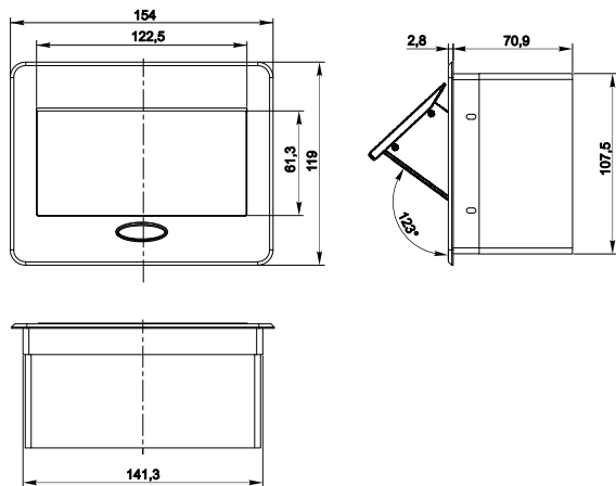
Рисунок 1 — Блок розеточный с выдвижной крышкой 4 модуля (PM-BR51-04-O-KXX)
