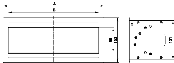
Рисунок 3 — Блок розеточный с односторонней крышкой
