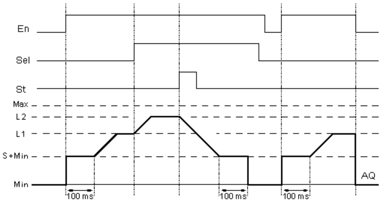
Временная диаграмма
