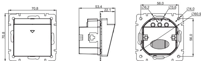
Рисунок 2 – Габаритные размеры выключателя / Figure 2 – Overall dimensions of switch / 2-сүрөт – Ажыраткыштың габариттй өлшемдөрй / Figura 2 – Dimensiunile generale ale întrerupătorului / ნახატი 2 – ამომრთველის გაბარითული ზომები / 2-сүрөт – Өчүргүчтүн көлөм өлчөмдөрү / Расми 2 – Андозай умумий калыдак / 2-rasm – Viklyuchatelning gabaritlari bo'yicha va o'rnatilish natijasidagi o'lchamlari
