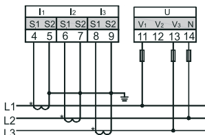
д) Трёхфазное, трёхпроводное подключение / Three-phase, three-wire connection / Үш фазалық, үш сымды жалғау (3P3W, 3-TT, 0-TH)
