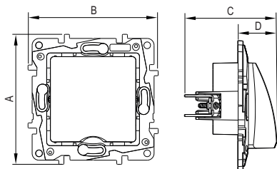
Рисунок 1 – Габаритные размеры вывода кабеля / Figure 1 – Overall dimensions of the cable outlet / 1 сурет – Кабель шықпасының габариттік өлшемдері / Figura 1 – Dimensiuni de gabarit ale ieșirii de cablu / 1-rasm – Kabel chiqargichning gabarit o'lchamlari
