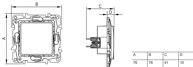
Рисунок 2 – Габаритные размеры адаптера / Figure 2 – Overall dimensions of the adapter / 2 сурет – Бейімдегіштің габариттік өлшемдері / Figura 2 – Dimensiuni de gabarit ale adaptorului / 2-rasm – Adapternig gabarit o'lchamlari
