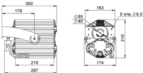
Рисунок 1 Общий вид светильника «L-lego II 110 banner» Поворотное крепление
